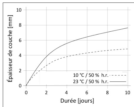
Diagramme 1: Vitesse de durcissement de Sikaflex®-521 UV
