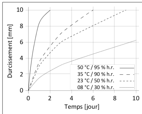
Diagram 1: Vitesse de polymérisation du Sikasil® SG-20
